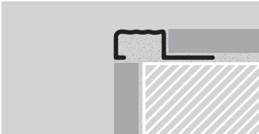
USO. Protege los escalones/gradas. USES. It protects steps/stands.
