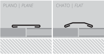
USO. Como divisor de pisos y alfombras. USE. As divider of floors and carpets.
